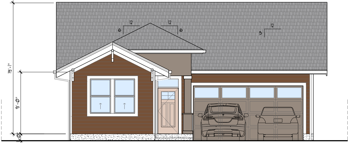
1266 ELEVATION R-A
