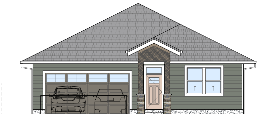
1480 - ELEV A
